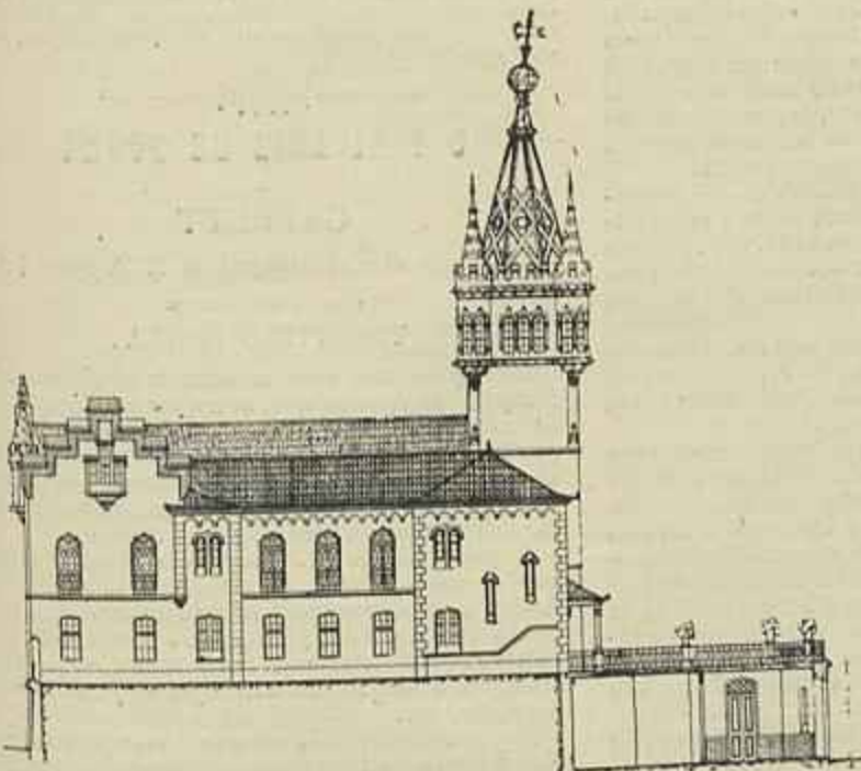
FACHADA POSTERIOR
