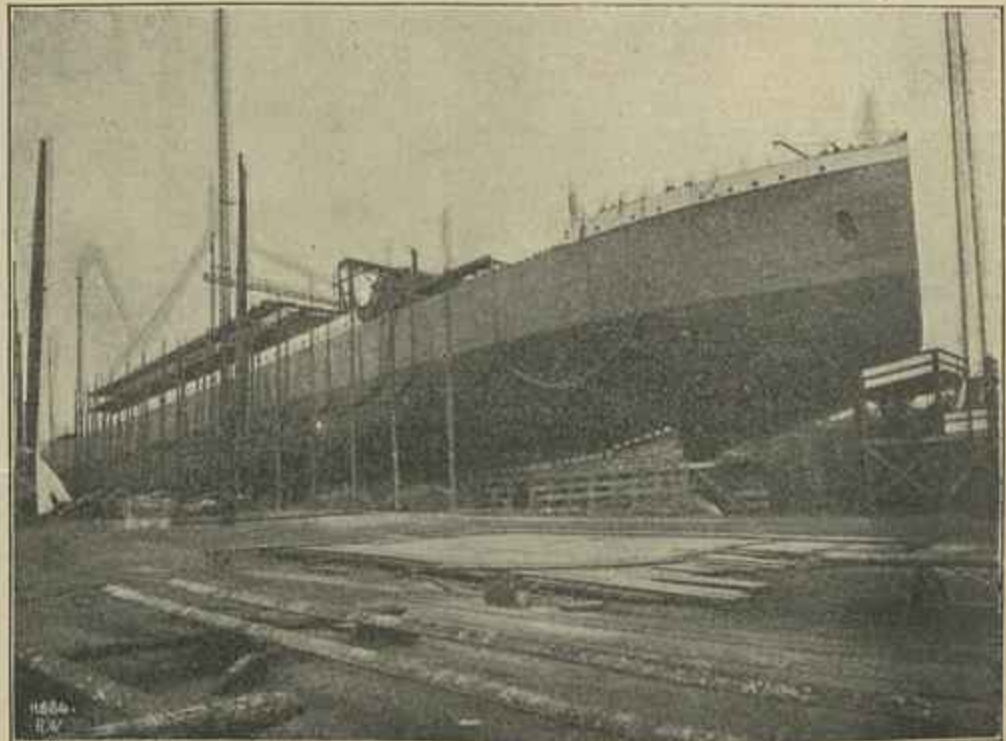
O "ARAGON", NO ESTALEIRO, VISTO DE PROA
