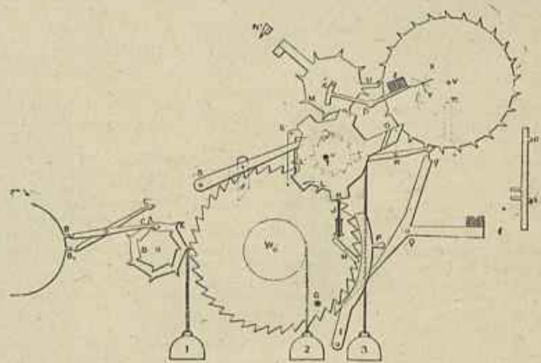
Fig. 22 — Schema do calendario mechanico
