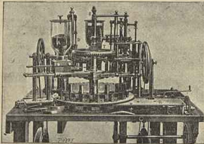
Fig. 20 — Machina para fabricar cartuchos de polvora para caça
