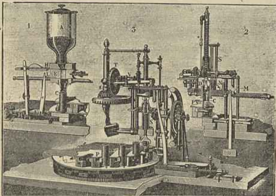
Fig. 21 — Detalhes da machina de fabricar cartuchos de polvora para caça
