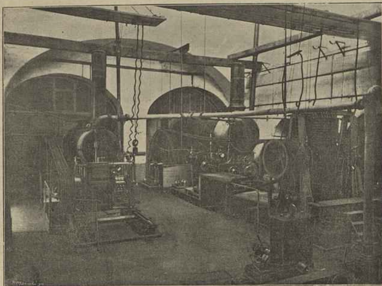
MACHINA DE VAPOR DE MARSHALL SONS & C.* DE 50 CAVALLOS E DYNAMO SIEMENS DE 36 KILOWATTS
