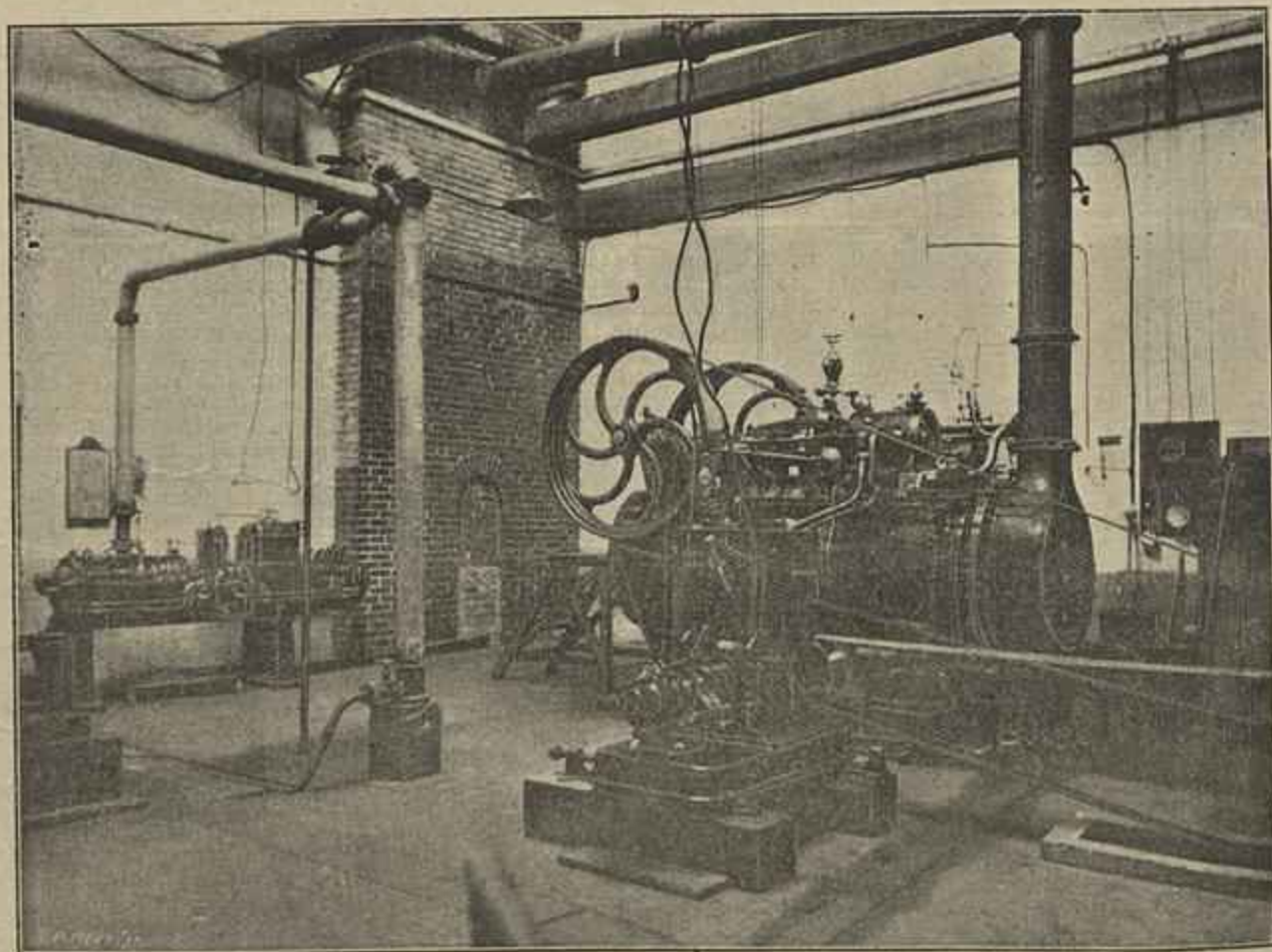
TURBINA A VAPOR E DYNAMO PARSON DE 18 KILOWATTS
