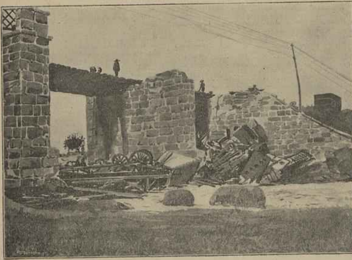
DESABAMENTO DA PONTE DE PAPA-GALLOS NO CAMINHO DE FERRO DO SUL
