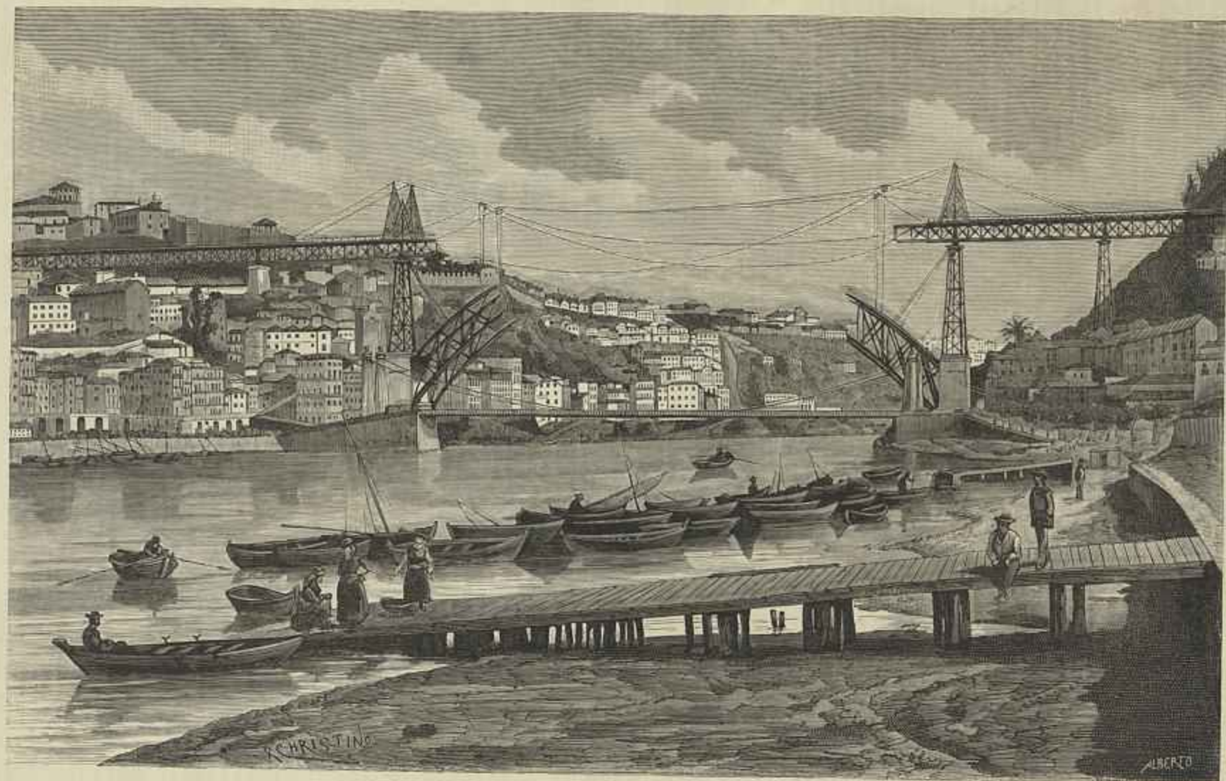
PONTE D. LUIZ I, NO PORTO. ESTADO ACTUAL DAS OBRAS (Segundo uma photographia de casa Eiel & C., do Porto)
