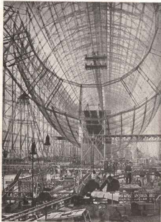
A carcassa do "Hindenburg" em construção nos estaleiros de Friedrichshafen
