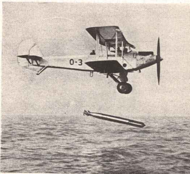
Um avião-torpedeiro largando o seu projectil
